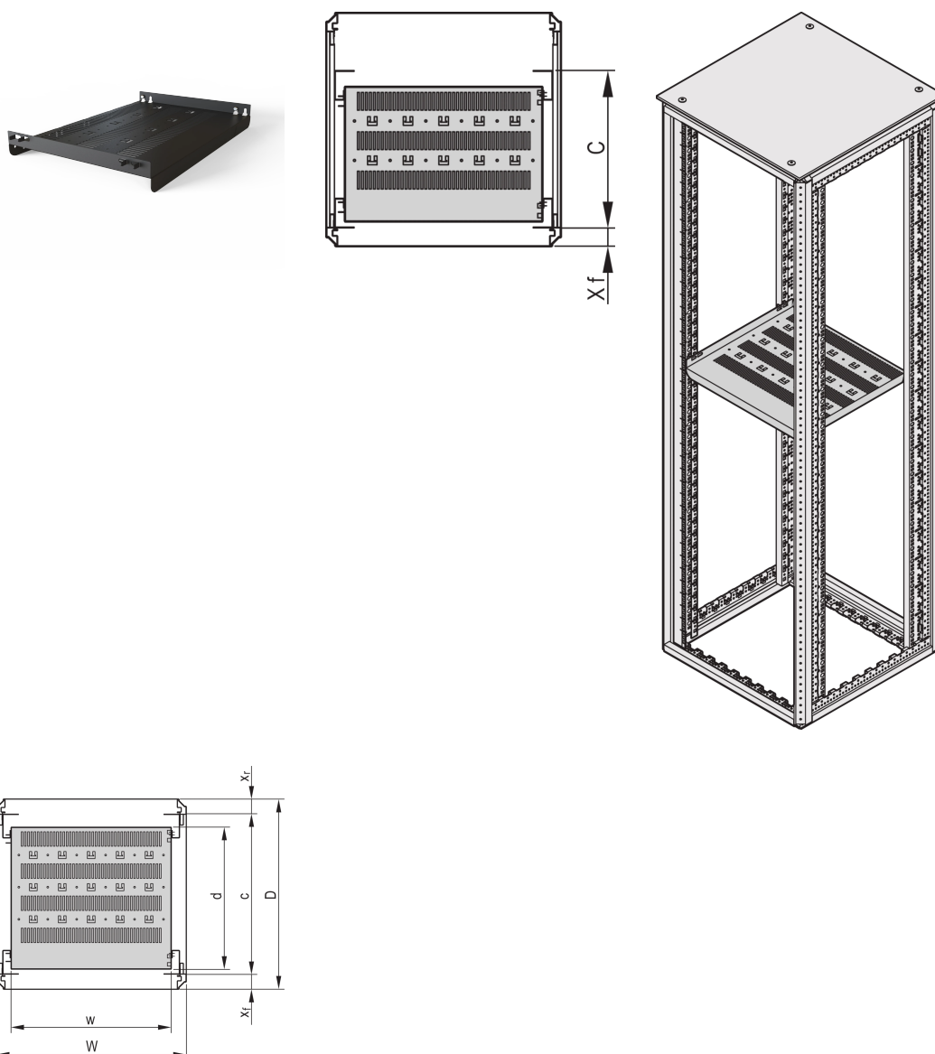
Varistar 19" Estantería, estacionaria, 75 kg.
