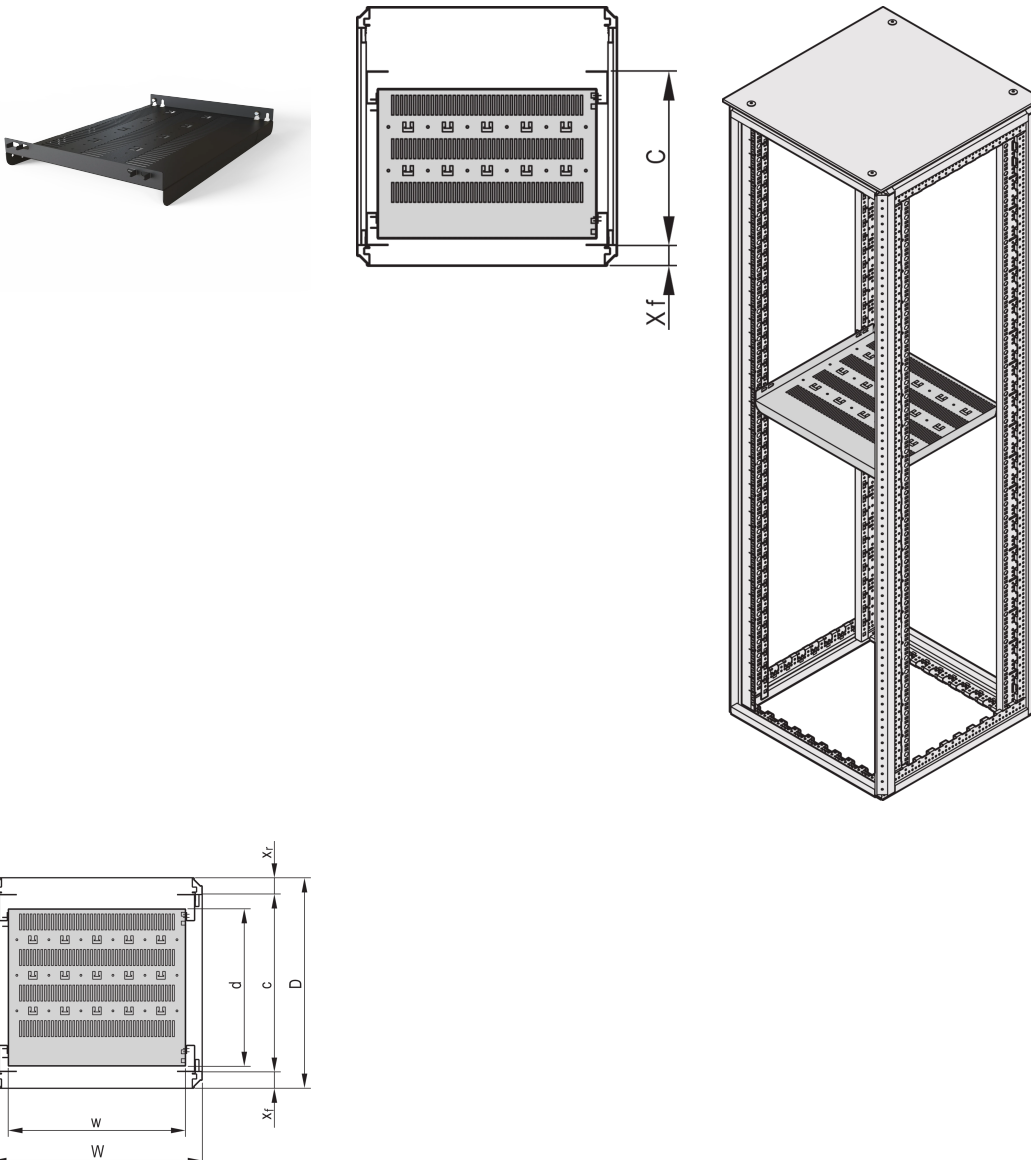
Étagère 19" Varistar, fixe, 75 kg.
