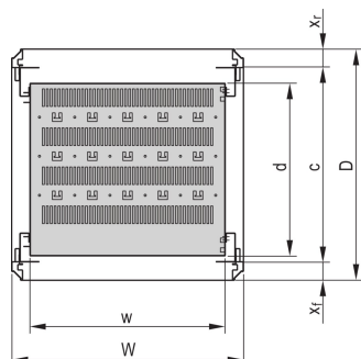
Półka Varistar 19", stacjonarna, 75 kg.
