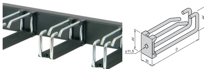
Gummiauflage montiert auf Doppel-Stahlkabelöse
