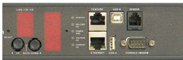
Display, Schnittstelle
