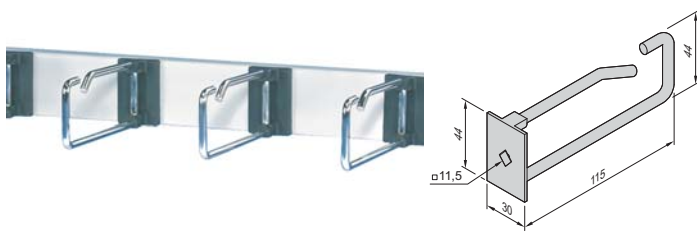
Stahlkabelöse auf 19"-Frontplatte montiert
