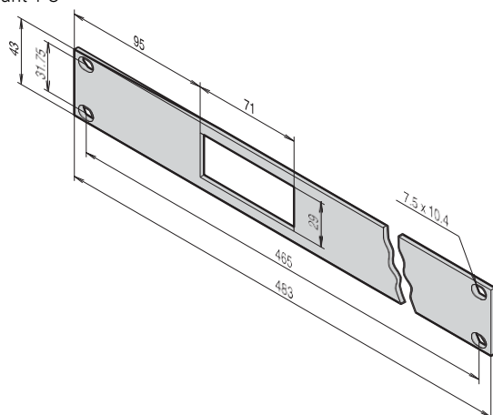
Face avant 1 U
