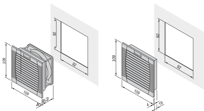
Ventilateur-filtre FL 100 Filtre d'entrée/sortie FLA 100
