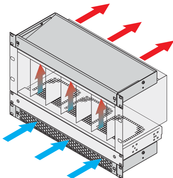
Guide d'air 1 U (inférieur) avec tiroir de ventilation 1 U (supérieur)
