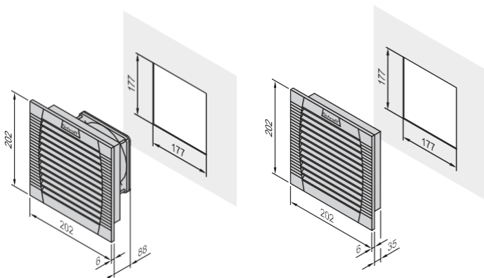
Filtre de rechange IP 54
