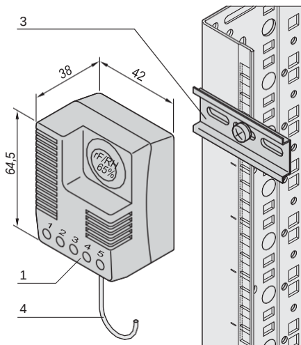
Hygrostat avec humidité relative réglable ou à réglage fixe
