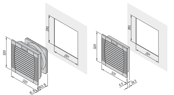
Ventilateur-filtre FL 500/600 Filtre d'entrée/sortie FLA 500/600 Tôle d'épaisseur 1 ... 2 mm - découpe 223 x 223 mm; Tôle d'épaisseur >2 ... 3 mm - découpe 224 x 224 mm
