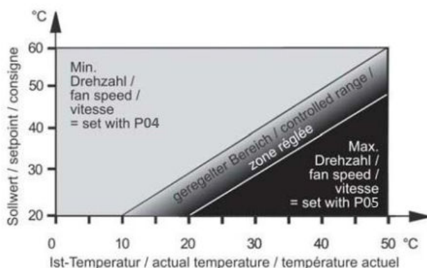
Régulation de la vitesse du ventilateur selon la température
