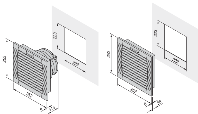
Filtre de rechange IP 54
