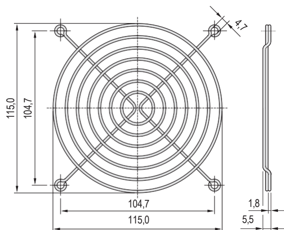
Grille de protection
