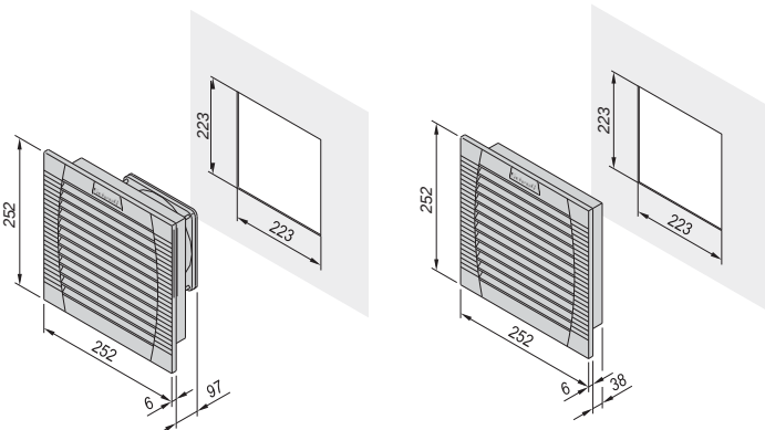
Ventilateur-filtre FL 250 Filtre d'entrée/sortie FLA 250/300 Tôle d'épaisseur 1 ... 2 mm - découpe 223 x 223 mm; Tôle d'épaisseur >2 ... 3 mm - découpe 224 x 224 mm
