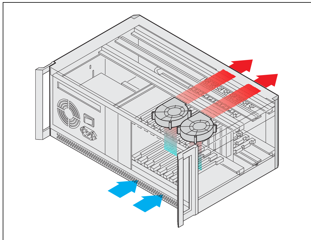
Figure 2: Entwärmung
