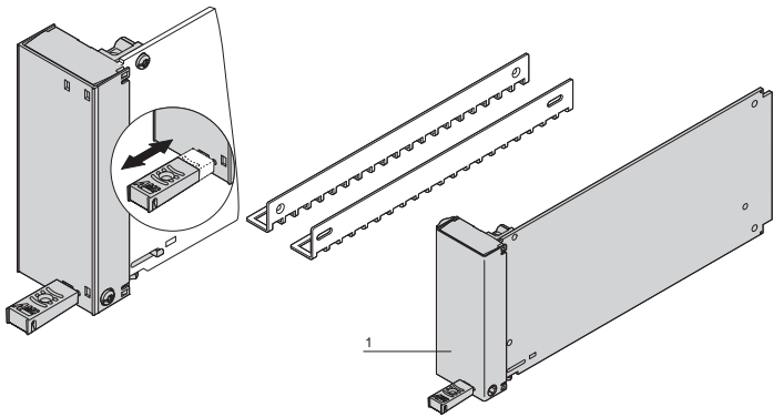
Pull-Griffmechanik
