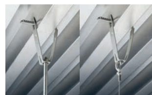
Tige filetée/chaîne/câble sur bac acier trapézoïdal
