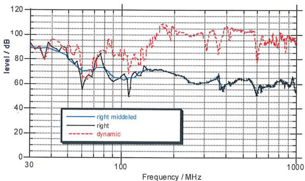
Abbildung 8: Messergebnisse bei direkter Einstrahlung auf die rechte Seitenwand
