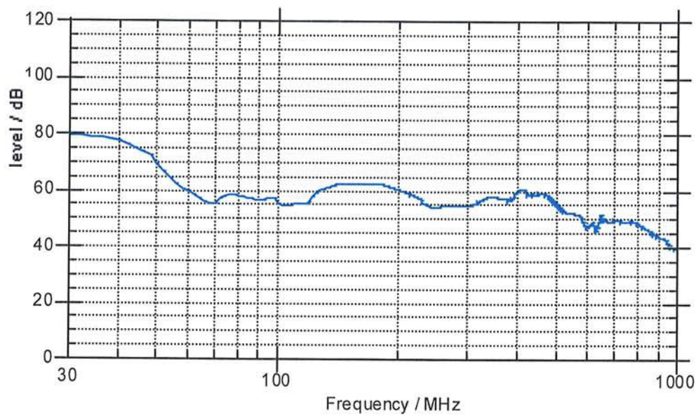
Abbildung 9: Typische Schirmdämpfung und Worst-Case-Abschätzung des Prüfobjekts
