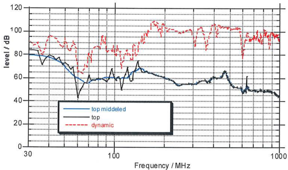
Abbildung 5: Messergebnisse bei direkter Einstrahlung auf die Obere-Seite des Prüfobjekts
