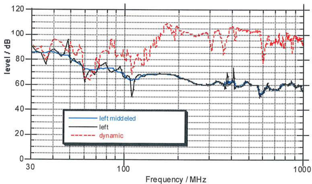
Abbildung 6: Messergebnisse bei direkter Einstrahlung auf die linke Seitenwand
