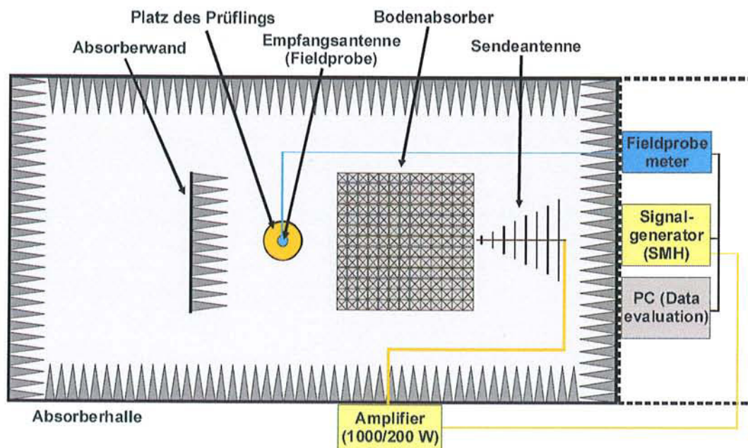
Abbildung 1: Messaufbau für Schirmdämpfungsmessungen
