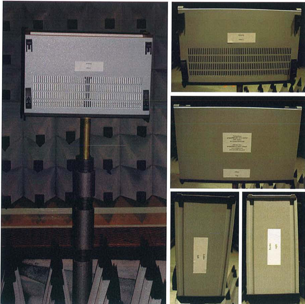
Abbildung 4: Prüfling am festgelegten Messplatz
