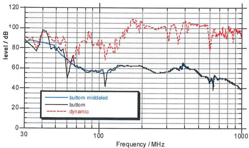
Abbildung 7: Messergebnisse bei direkter Einstrahlung auf die Untere-Seite des Prüfobjets
